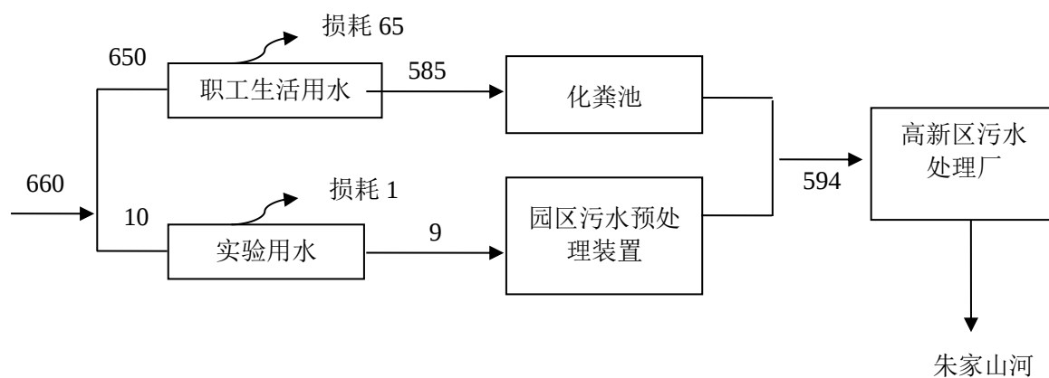
图 2-1 建设项目用水平衡图 (t/a)
