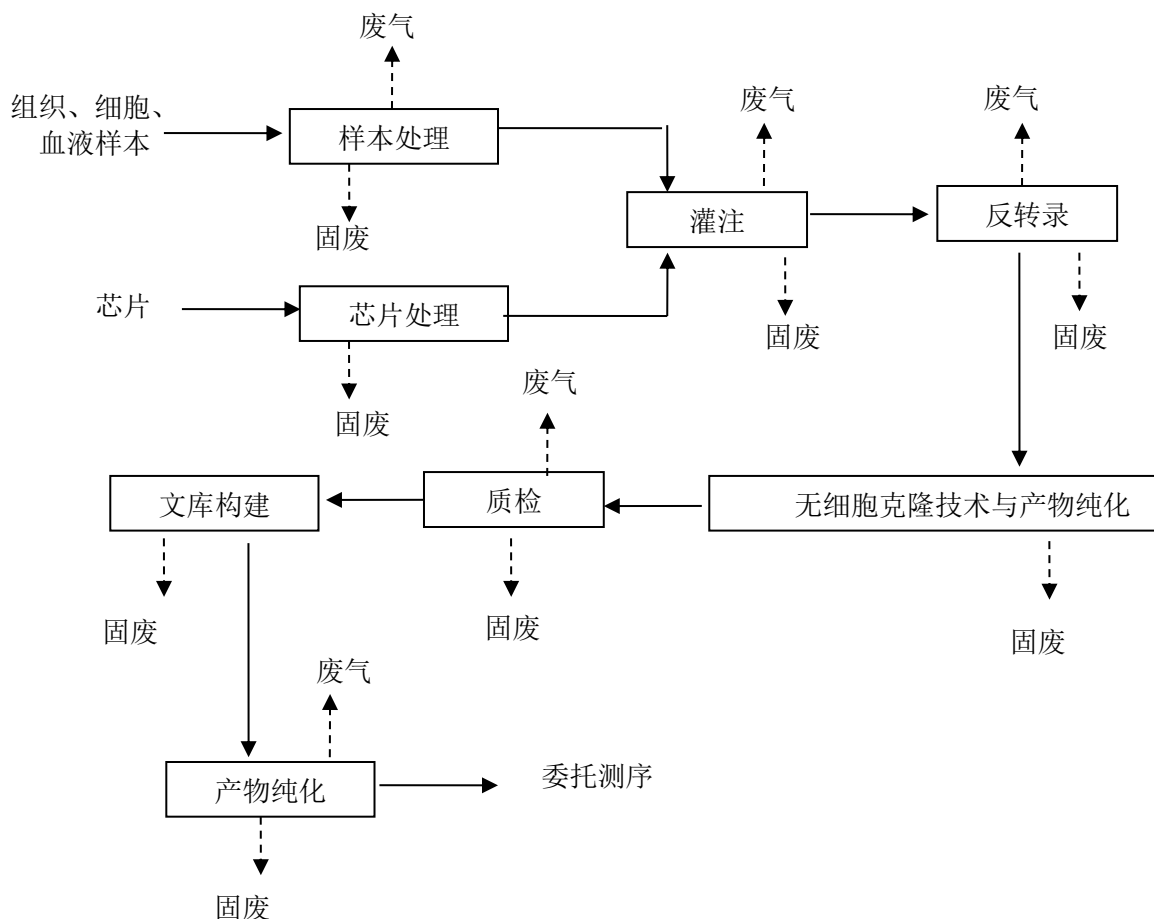
图 2-2 项目工艺流程及产污环节图
