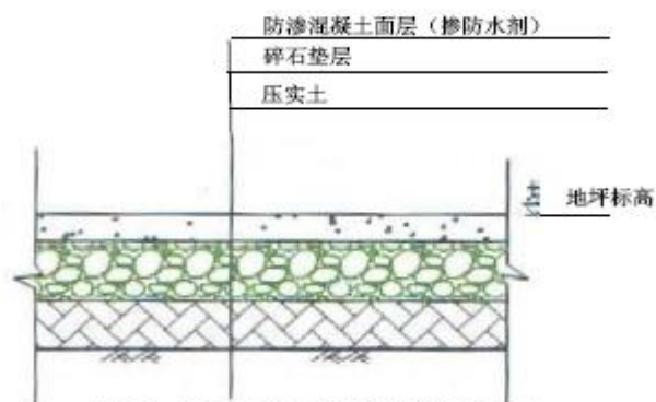
图 6.5-2 一般防渗区地面防渗结构图
