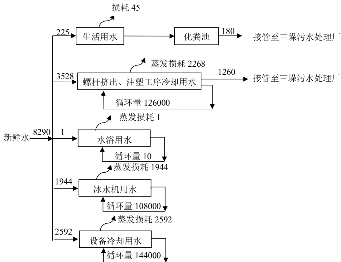
图 3.3-3 拟建项目水平衡图 单位： \text{m}^3/\text{a}
