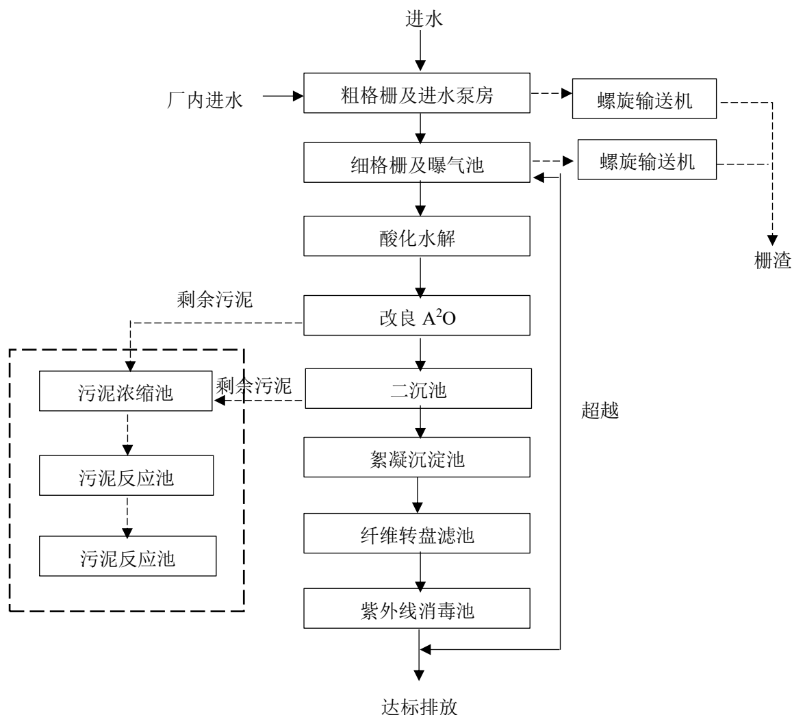
图 6.1-1 三垛镇（区域）污水处理厂三期污水处理工艺图
