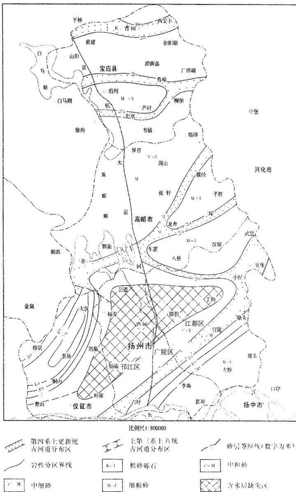
图4.1-1扬州市主要承压含水层水文地质分布图
