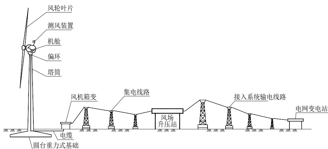
图 5-2 营运期主要工艺流程图
