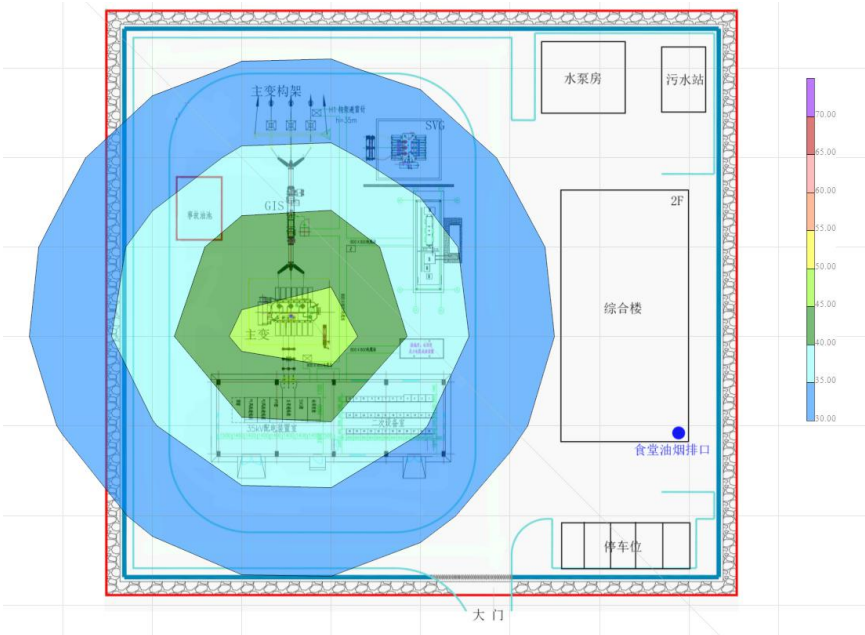
图 7-1 本项目升压站变压器噪声影响包络线图
