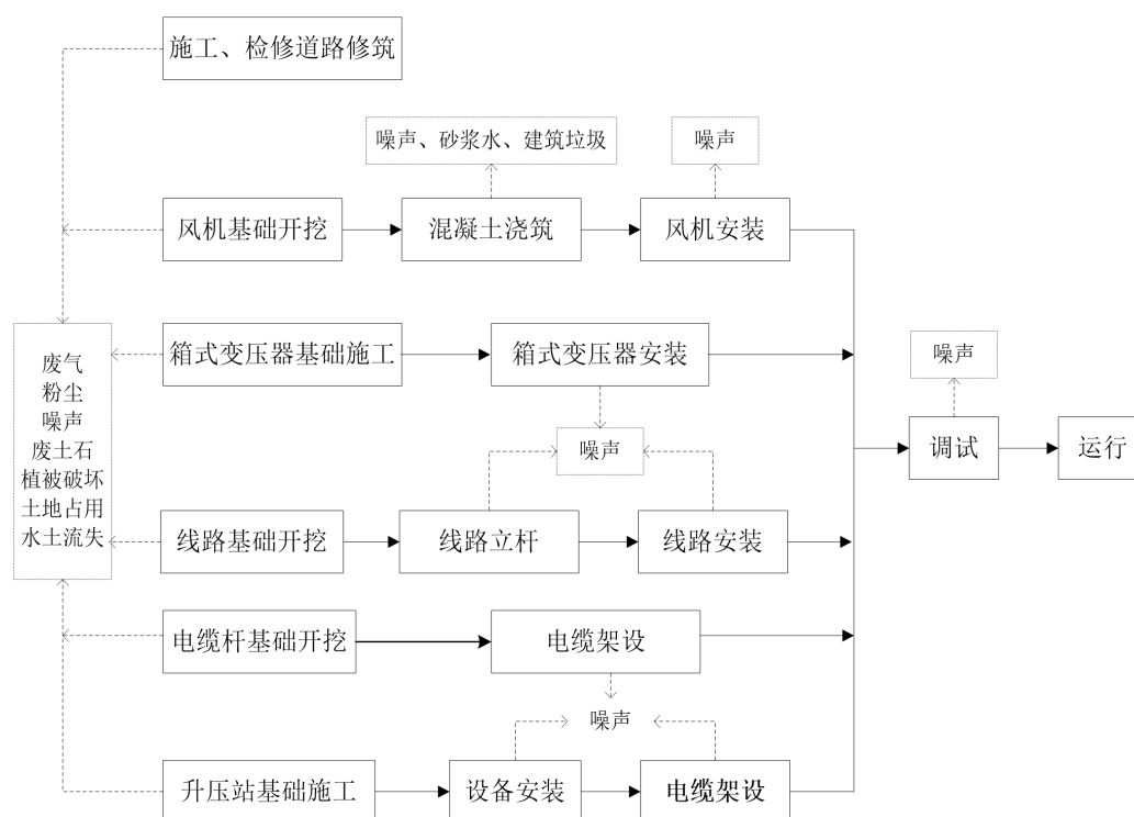
图 5-1 施工期主要工艺流程及产污环节示意图
