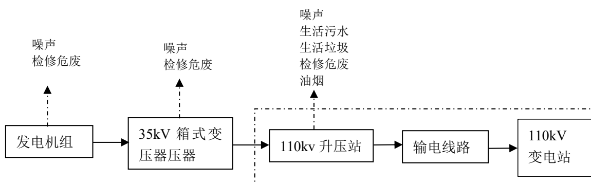
图 5-3 运营期产污环节图
