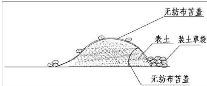
图 8-2 施工采取的临时苫盖措施示意图
