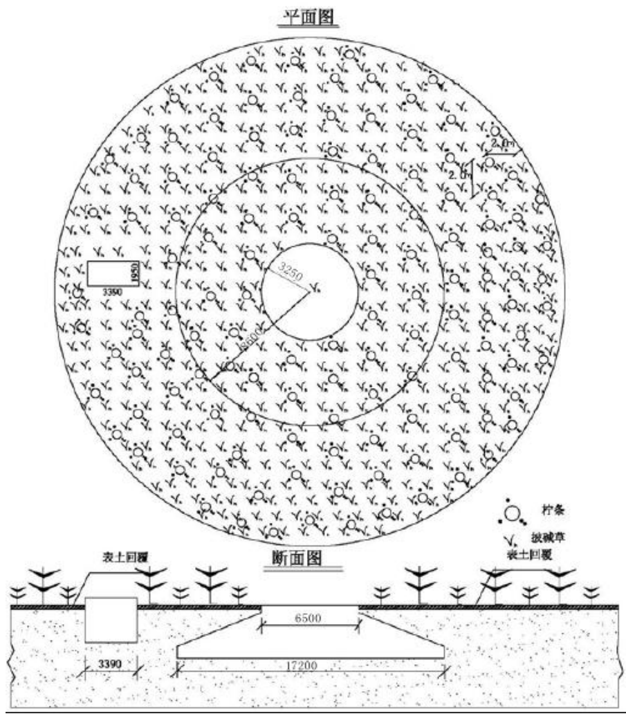
图 8-1 风机和箱式变基础典型生态保护措施布置示意图
