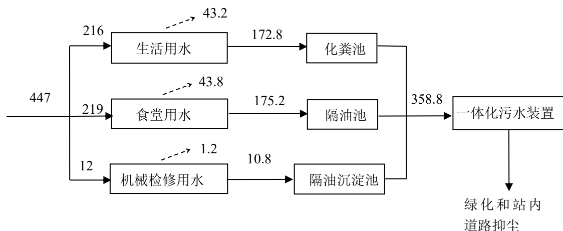
图 5-4 本项目水平衡图
