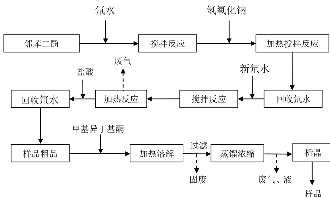
图 1 邻苯二酚-D4 研发工艺流程及产物环节图
