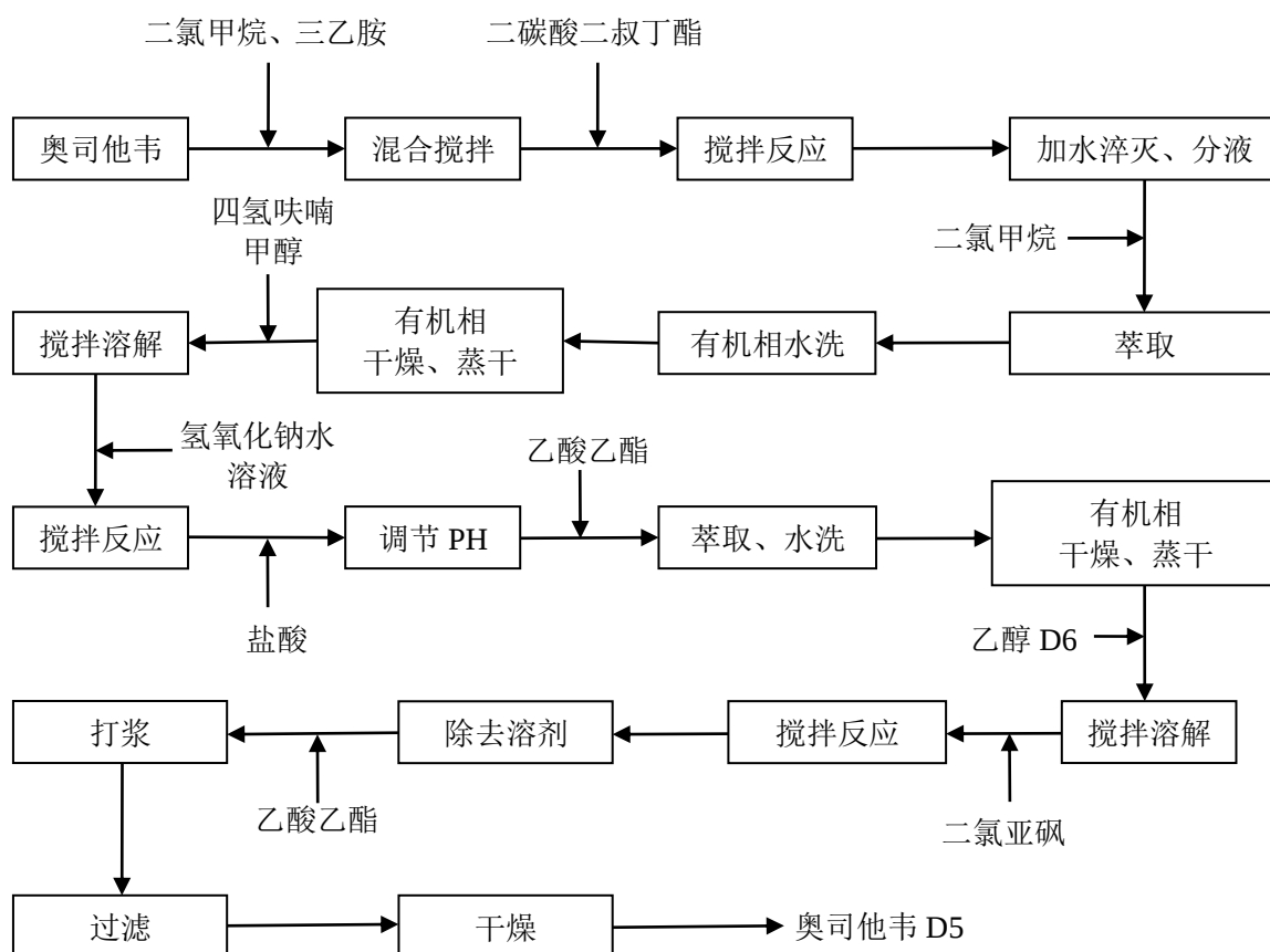
图 2 奥司他韦-D6 研发工艺流程及产物环节图
