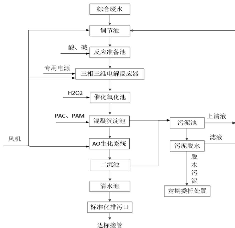
图 5 园区废水预处理工艺流程图
