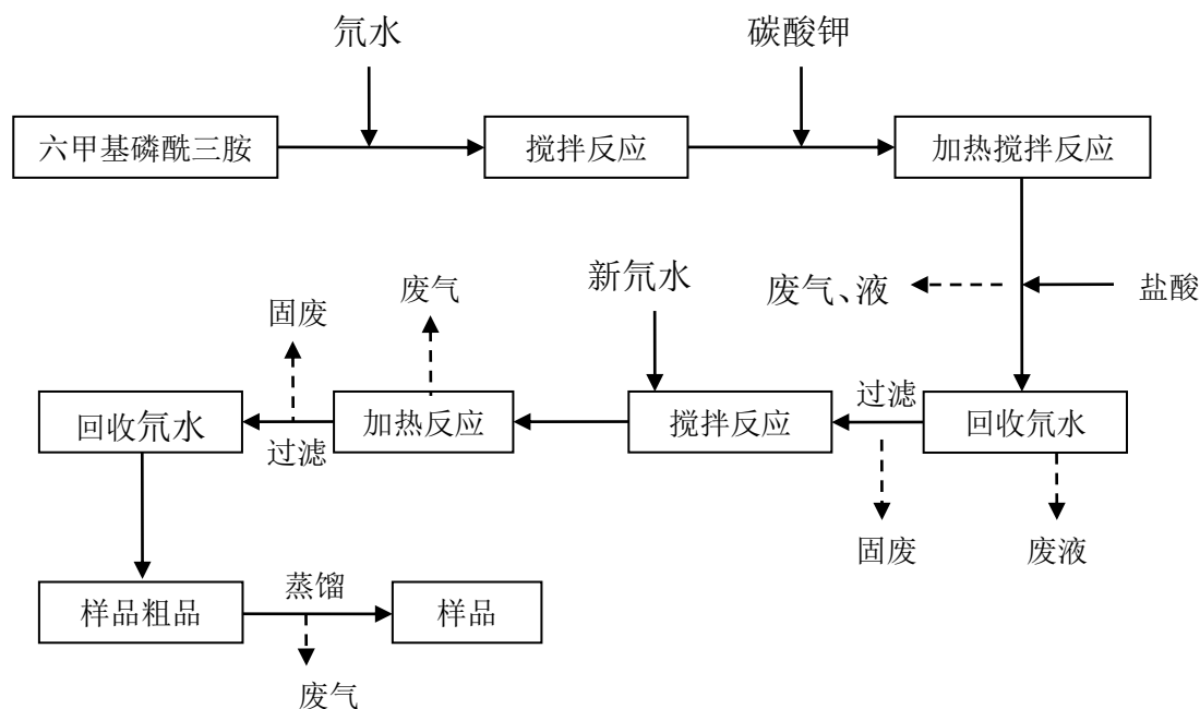
图 3 HMPA（六甲基磷酰三胺）-D18 研发工艺流程及产物环节图
