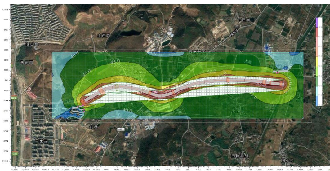
图 7-6 近期（2023 年）夜间交通噪声贡献值等值线图
