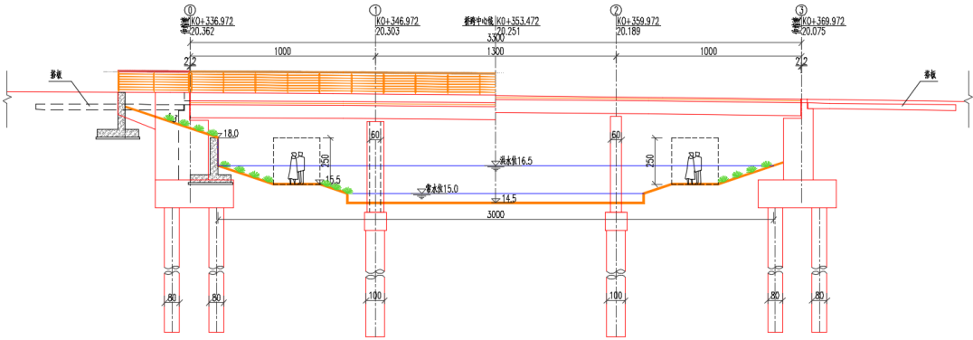
图 1-6 立面图（四清河桥）
