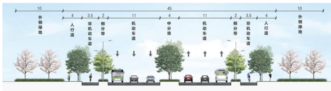
图 1-5 本项目道路横断面示意图
