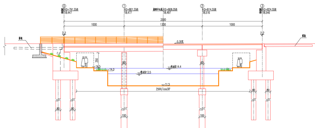
图 1-8 立面图（凤池河桥）
