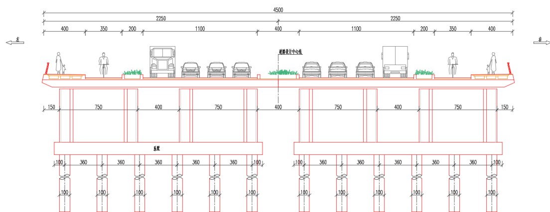
图 1-9 断面图（凤池河桥）
