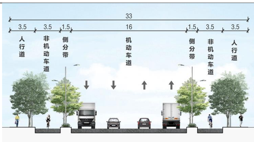
图 1-3 项目现状交叉断面图
