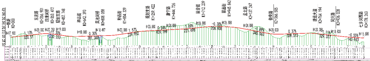
图1-4 项目设计道路纵断面设计图
