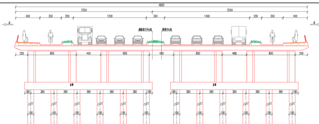
图 1-7 断面图（四清河桥）
