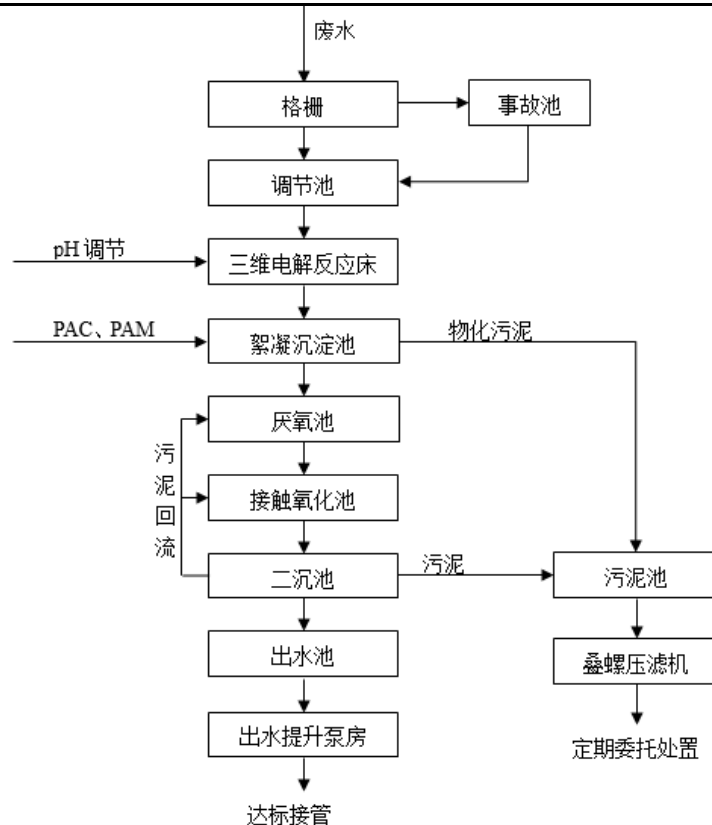
图 4-2 园区废水预处理工艺流程图
