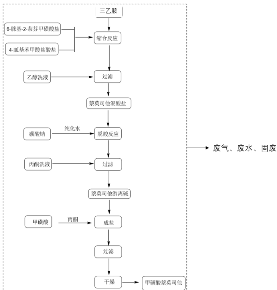
图 2-2 甲磺酸萘莫司他工艺流程
