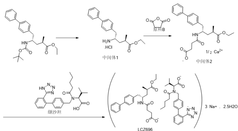
图 2-5 LCZ696 反应原理
