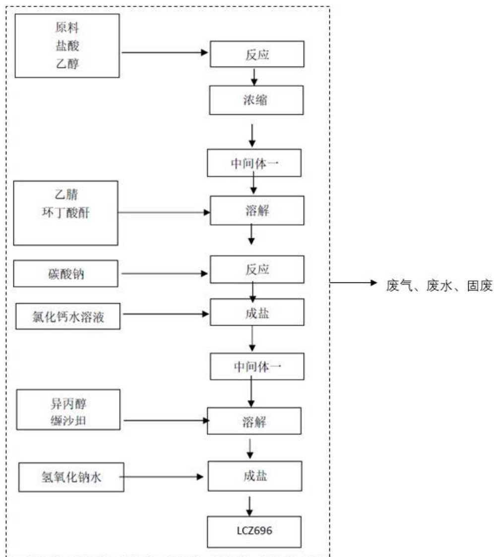
图 2-6 LCZ696 研发流程
