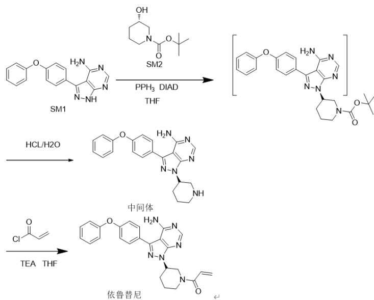
图 2-3 依鲁替尼反应原理
