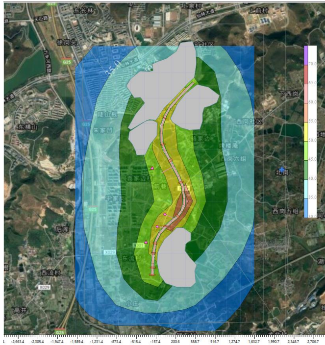
图 4-9 近期（2024 年）昼间交通噪声贡献值等值线图
