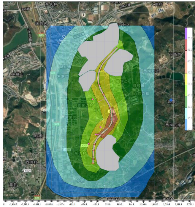
图 4-11 中期（2030 年）昼间交通噪声贡献值等值线图
