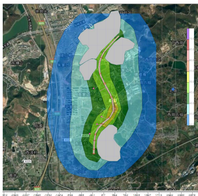
图 4-14 远期（2038 年）夜间交通噪声贡献值等值线图
