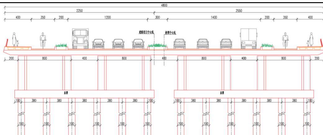
图 2-8 断面图（小白沟桥）
