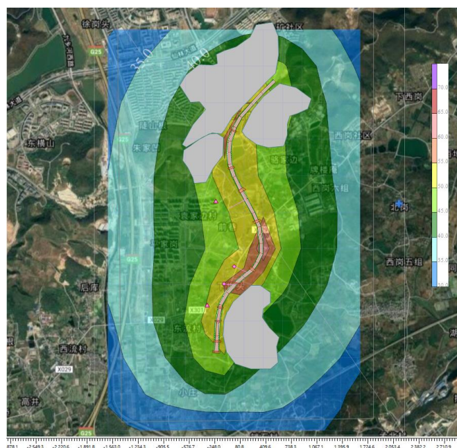
图 4-13 远期（2038 年）昼间交通噪声贡献值等值线图
