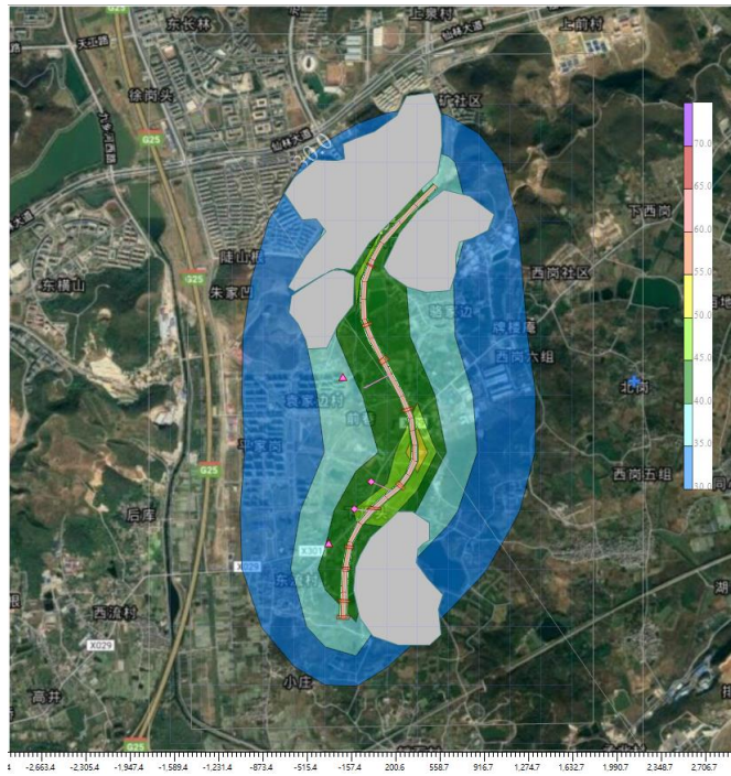
图 4-10 近期（2024 年）夜间交通噪声贡献值等值线图
