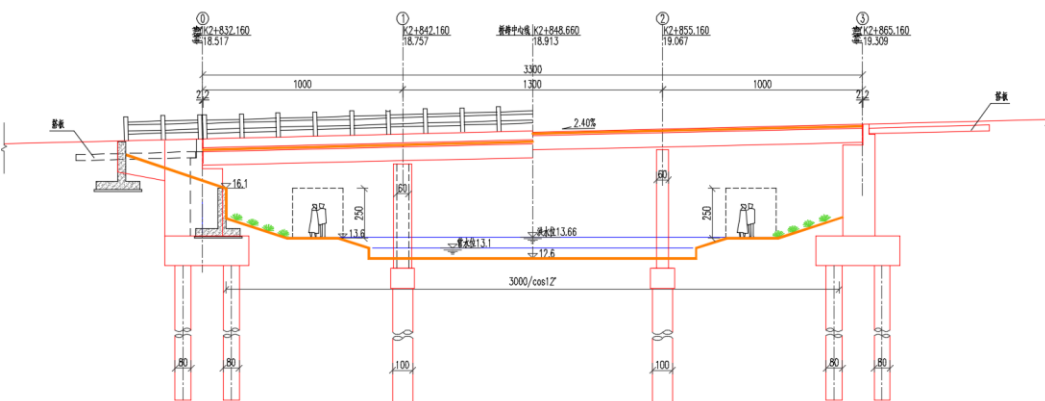
图 2-7 立面图（小白沟桥）
