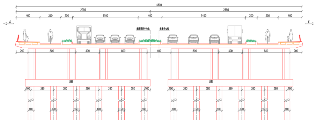
图 2-6 断面图（西袁河桥）
