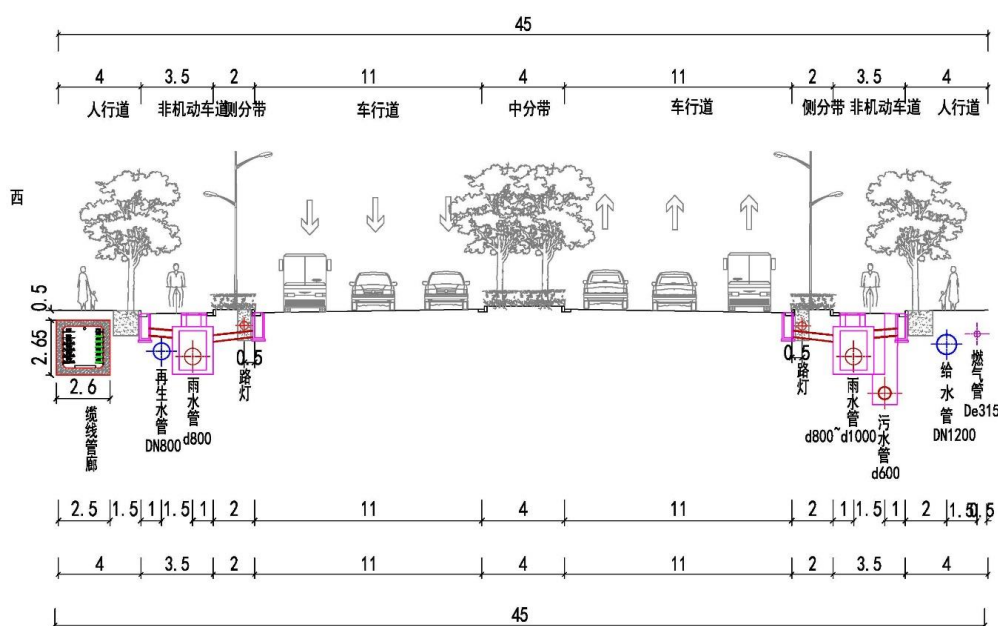
图 2-10 管线综合横断面设计图
