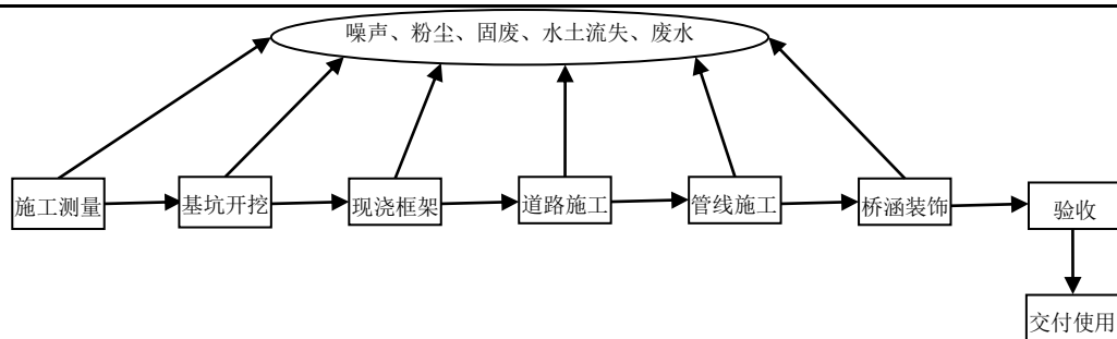
图 2-12 本项目桥梁工程及配套设施施工工艺流程及产污环节图
