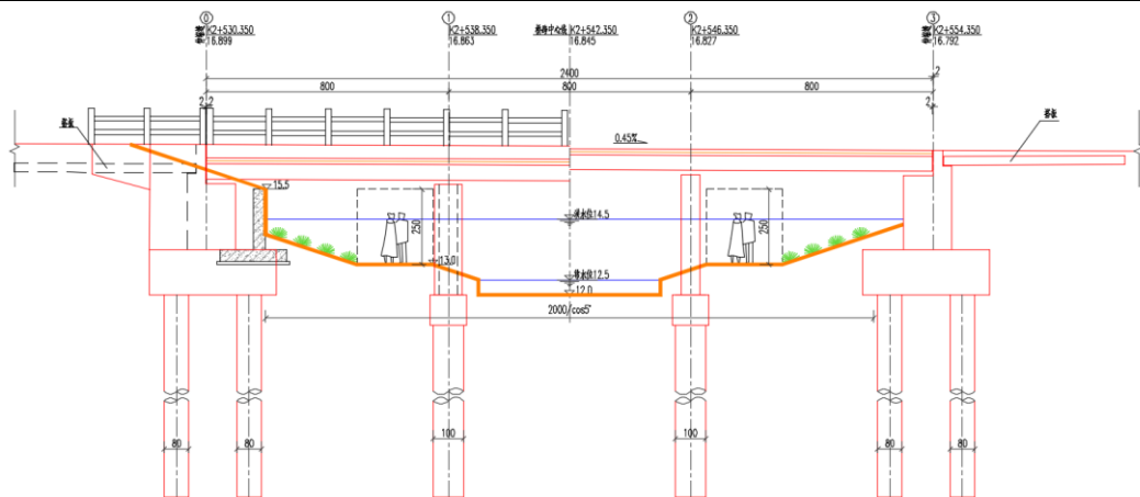
图 2-5 立面图（西袁河桥）
