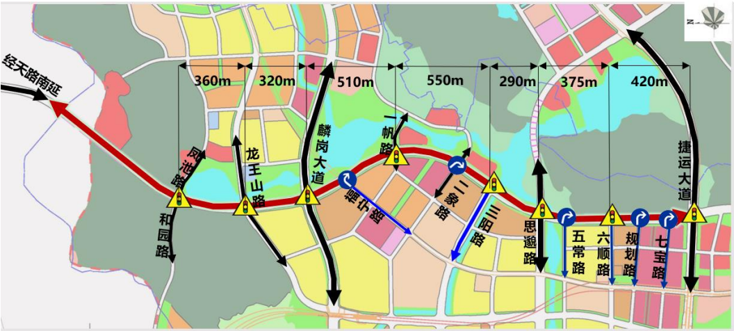
图 2-4 本项目道路交叉口示意图
