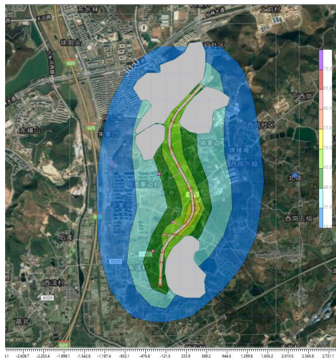
图 4-12 中期（2030 年）夜间交通噪声贡献值等值线图
