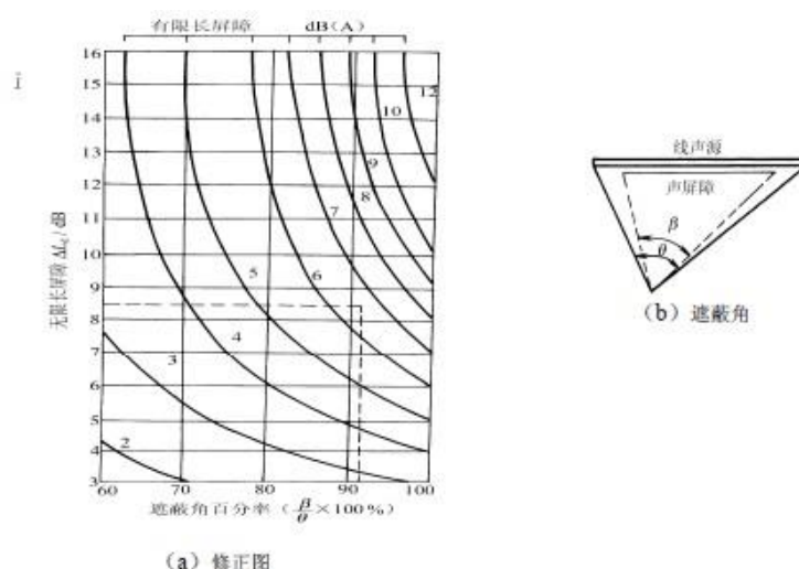
图 4-2 有限长度的声屏障及声源的修正图
