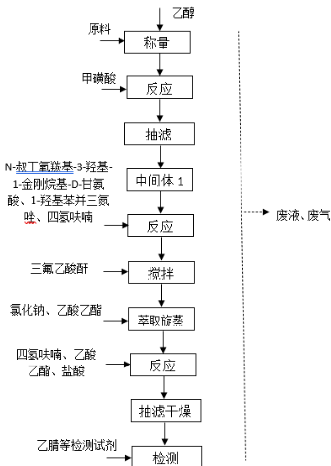
图2-3沙格列汀的研发工艺流程
