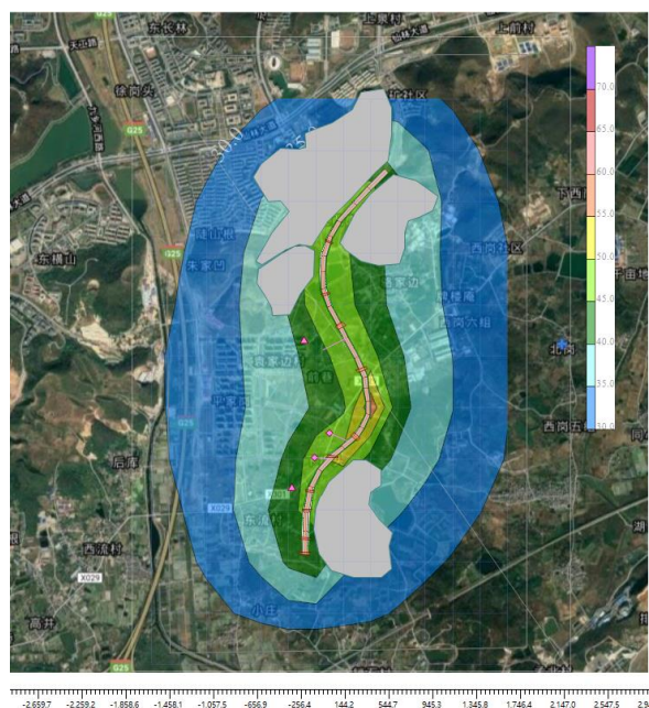
图 4-14 远期（2038 年）夜间交通噪声贡献值等值线图
