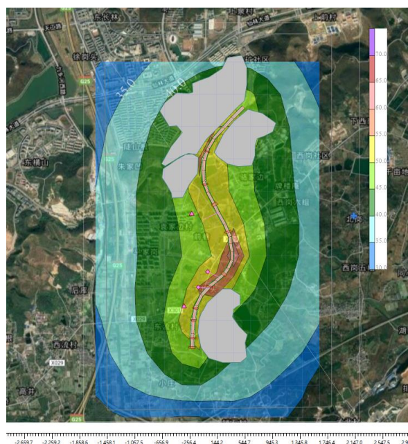
图 4-13 远期（2038 年）昼间交通噪声贡献值等值线图
