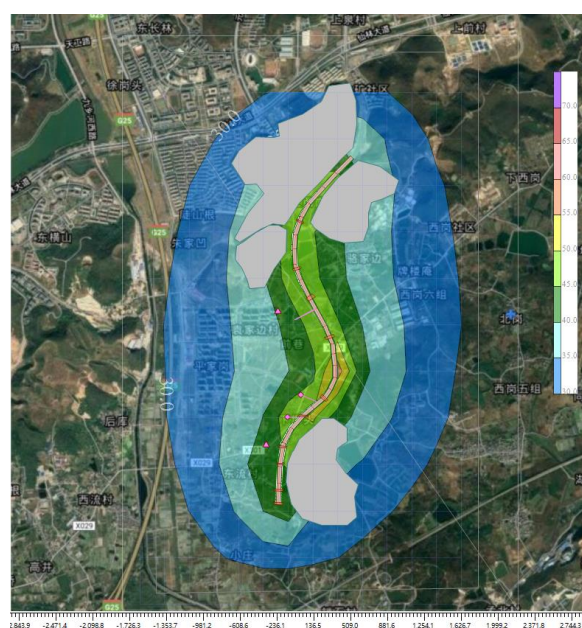
图 4-12 中期（2030 年）夜间交通噪声贡献值等值线图
